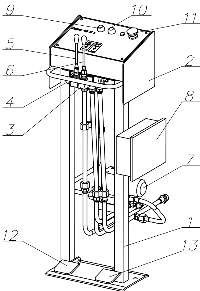
Рис. 6. Пульт управления.
